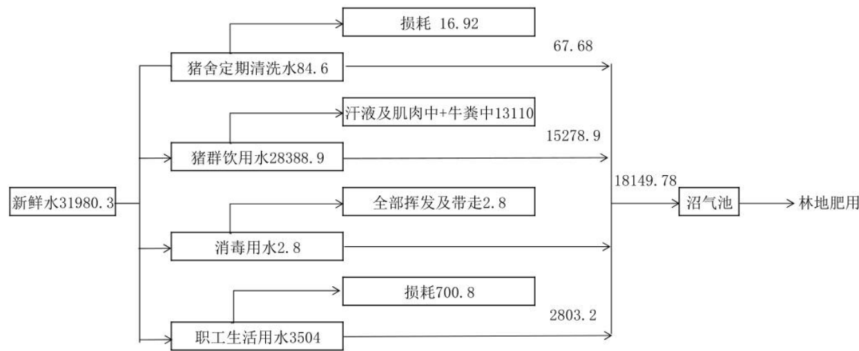
图 3.3-1 本项目水平衡图（t/a）
