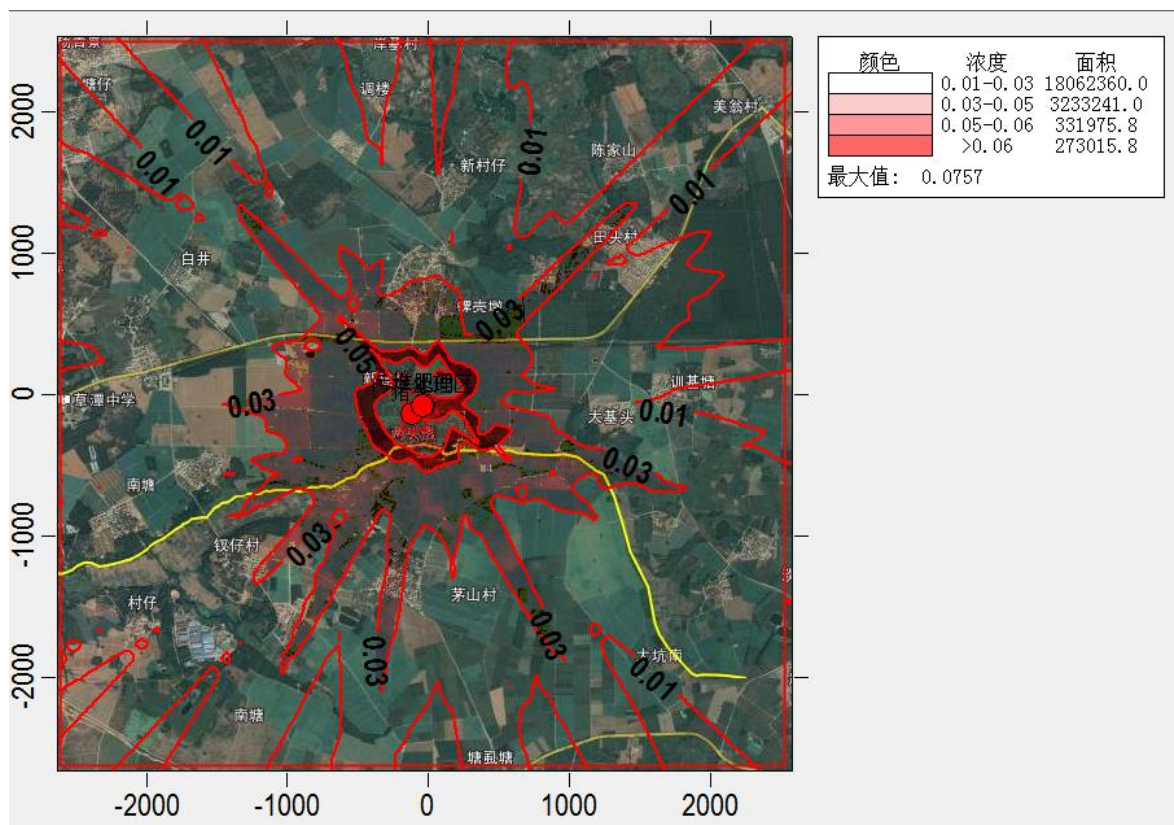
图 5.2-8 敏感点和最大落地浓度点 \text{NH}_3 1h 预测浓度
