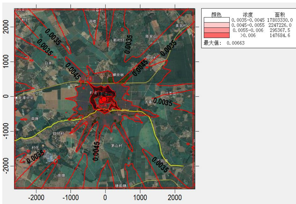
图 5.2-11 敏感点 H 2 S 1h 预测浓度叠加背景值
