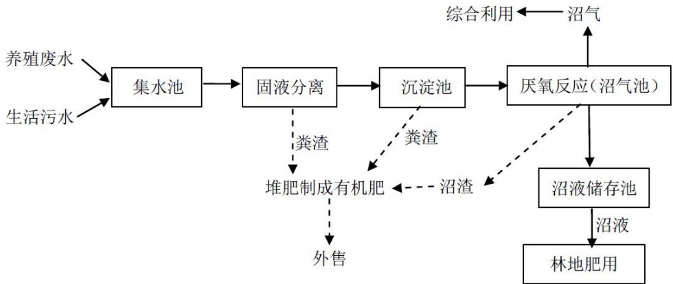
图 7.1-1 污水处理工艺流程图
