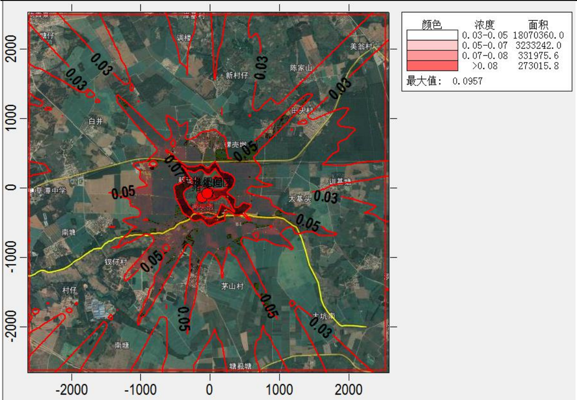
图 5.2-9 敏感点 \text{NH}_3 1h 预测浓度叠加背景值
