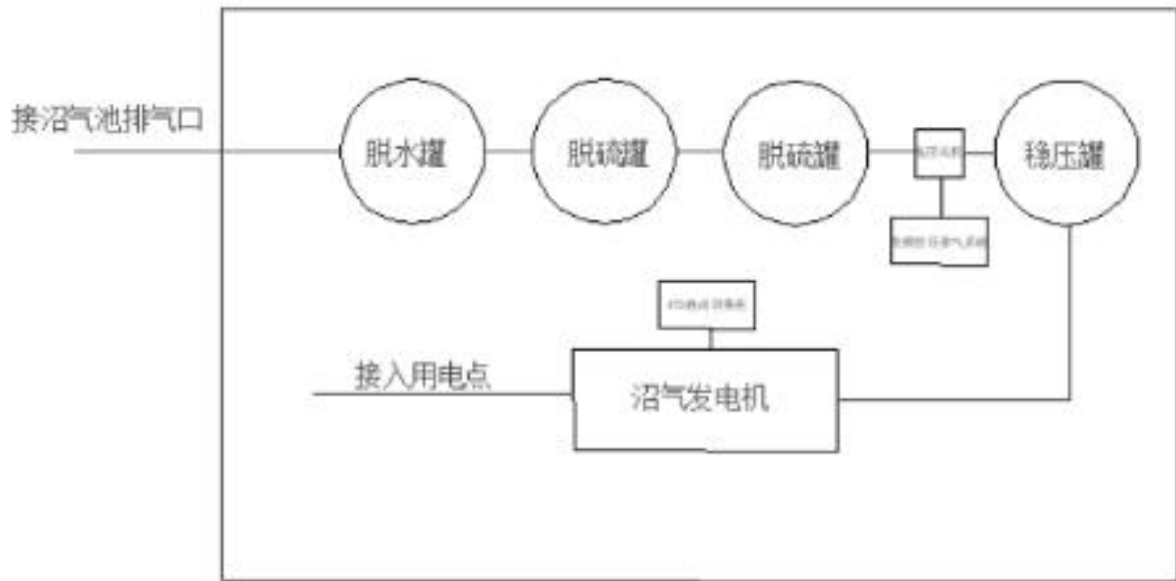
图 3.5-3 沼气发电系统流程图
