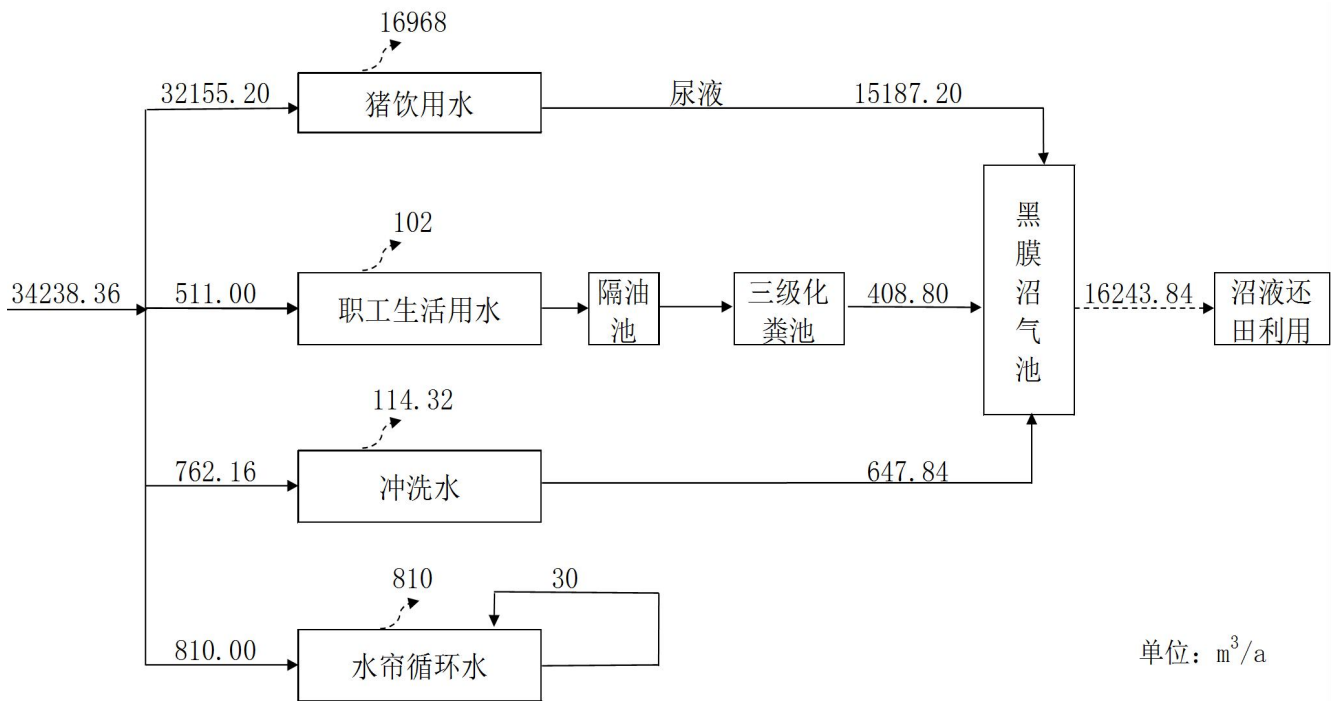
图 3.4-1 本项目水平衡图
