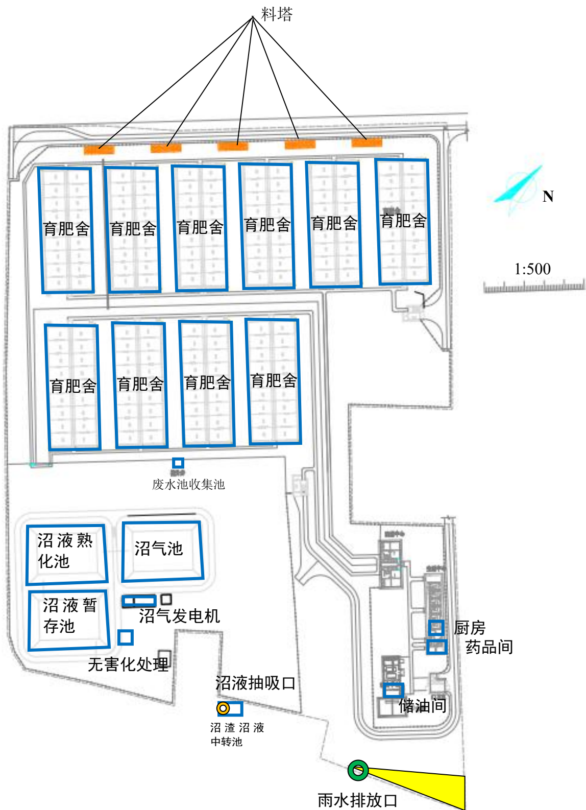
图 3-2 猪场平面布置图
