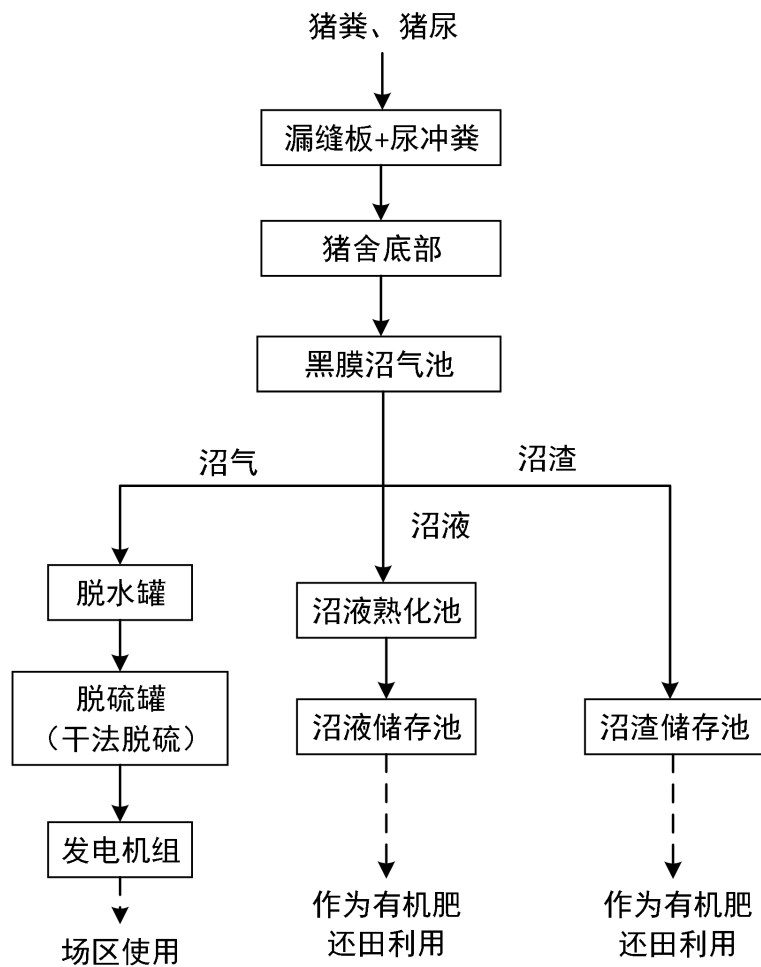
图 3-5 粪污处理及综合利用工艺图
