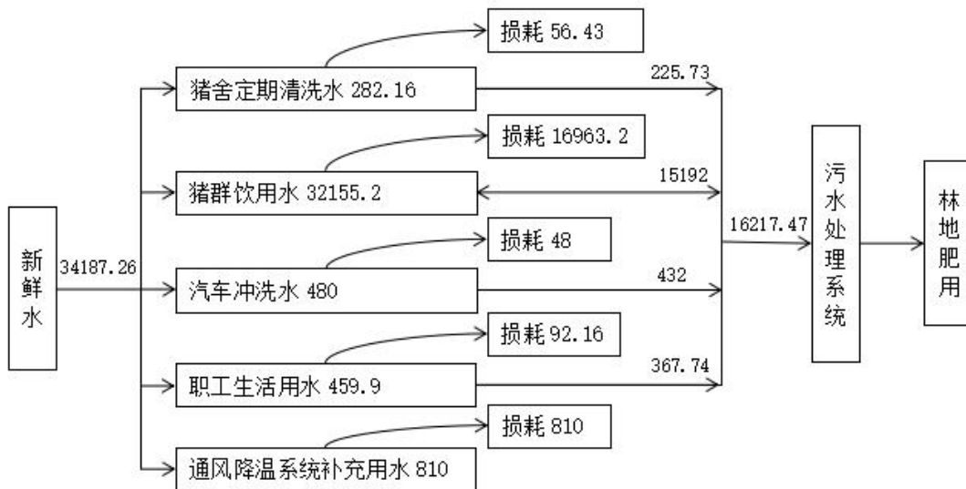
图 3-3 本项目水平衡图
