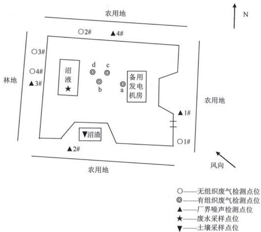
图 7-1 监测布点图
