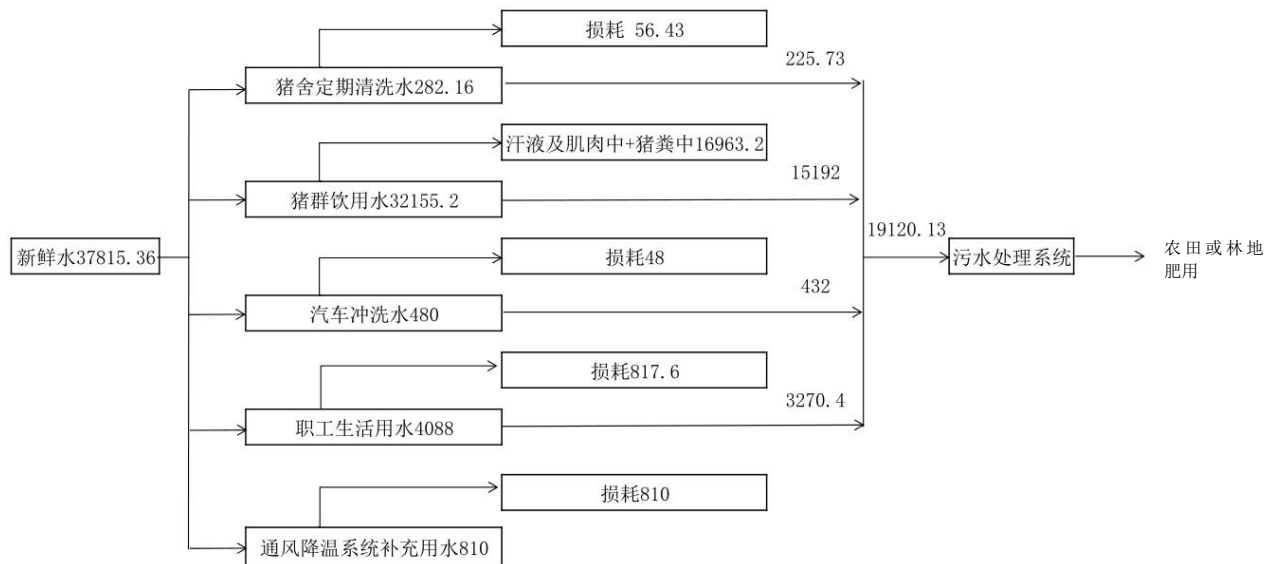
图 3.4-1 本项目水平衡图
