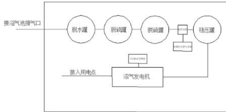
图 3.5-3 沼气发电系统流程图
