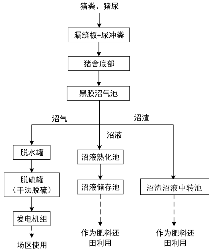
图 3-5 粪污处理及综合利用工艺图
