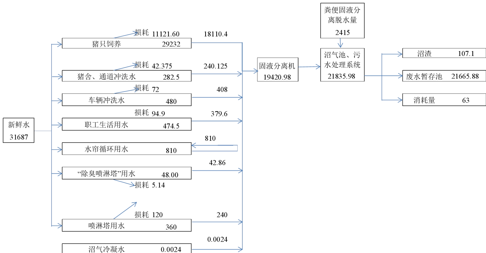
图 3-3 本项目水平衡图（单位： \text{m}^3/\text{a} ）
