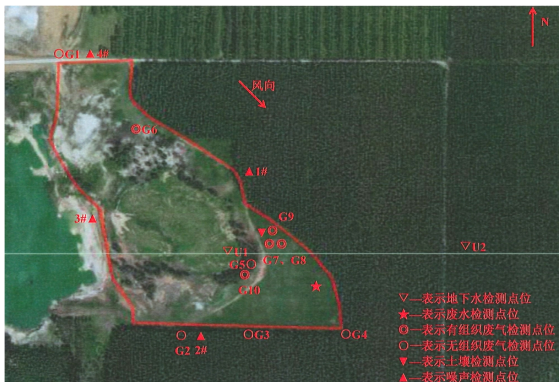
图 7-1 监测布点图
