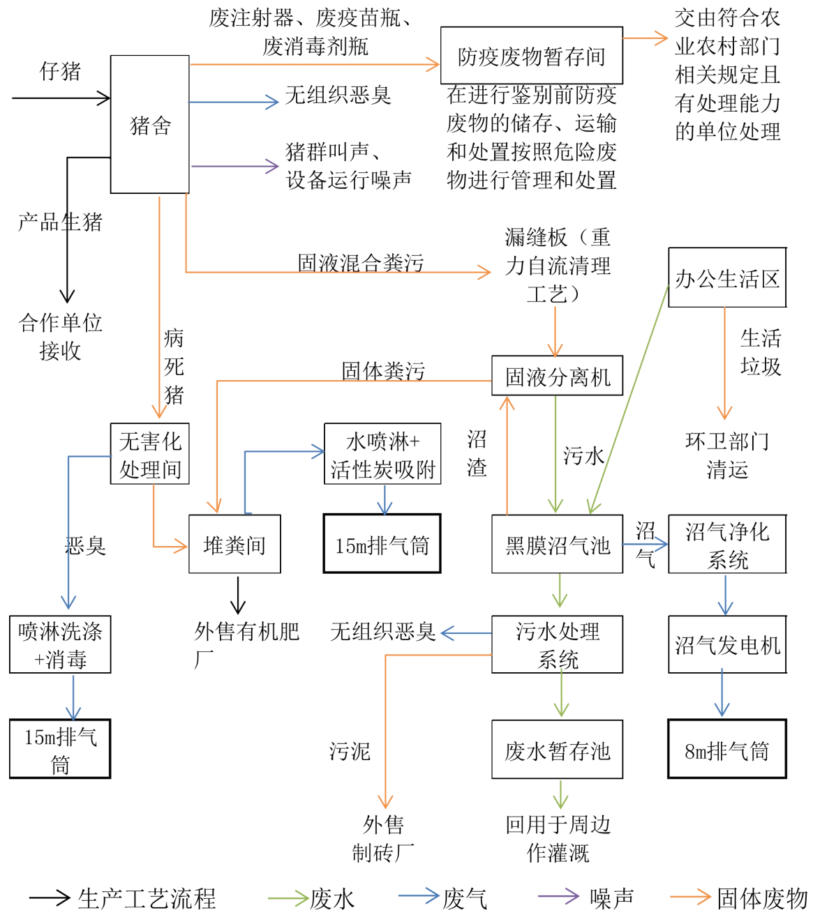
图 3-4 生产工艺流程图
