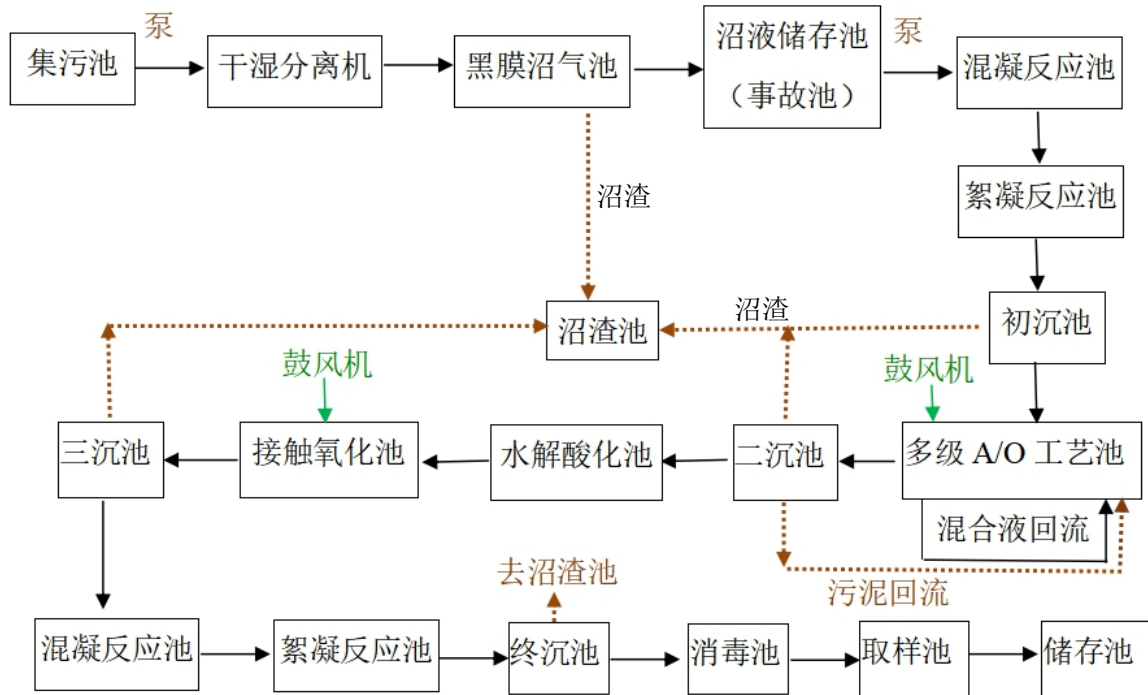
图 3-5 污水处理工艺示意图
