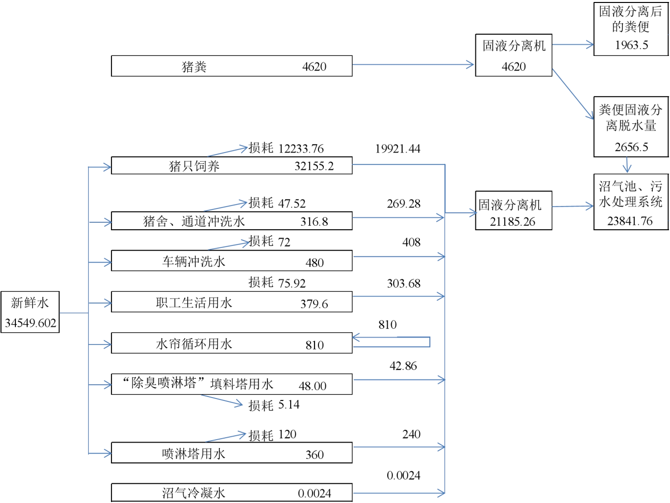
图 3-3 本项目水平衡图（单位：m³/a）
