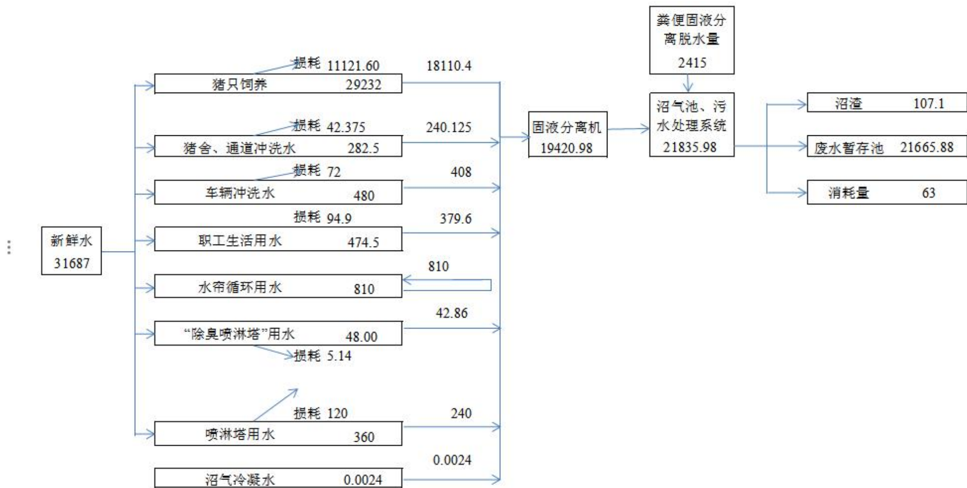
图 3-3 本项目水平衡图（单位： \text{m}^3/\text{a} ）
