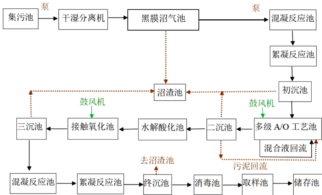
图 3-5 污水处理工艺示意图
