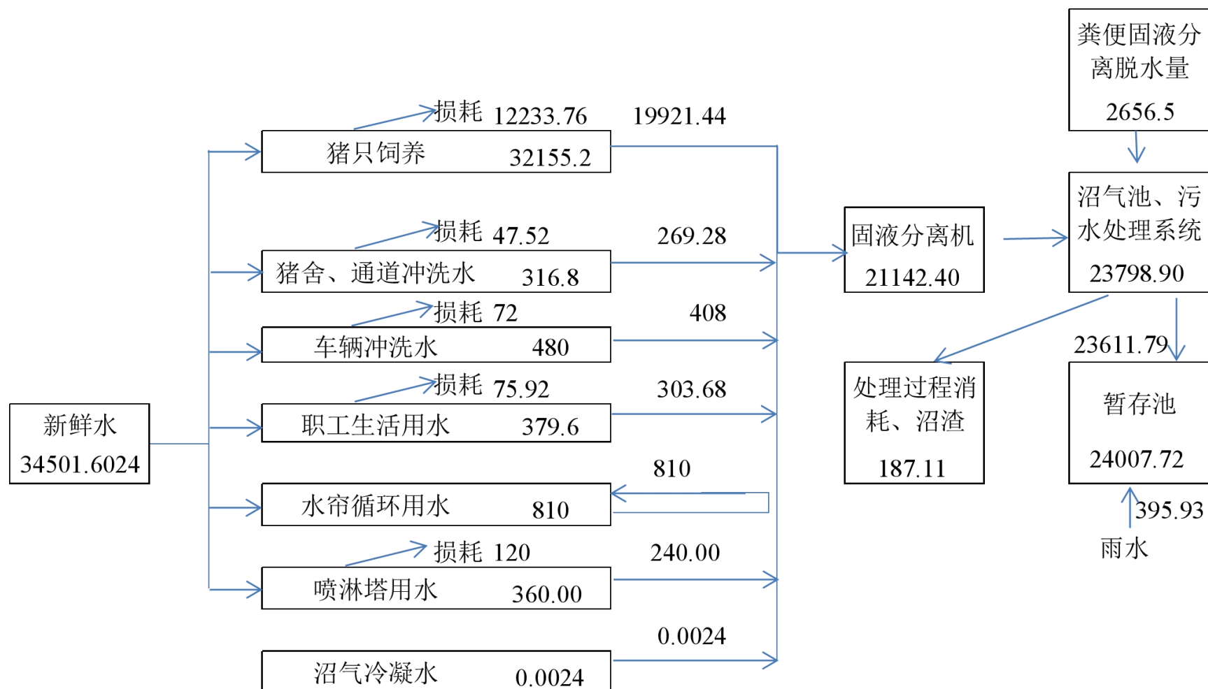
图 3-3 本项目水平衡图 (单位: \text{m}^3/\text{a} )
